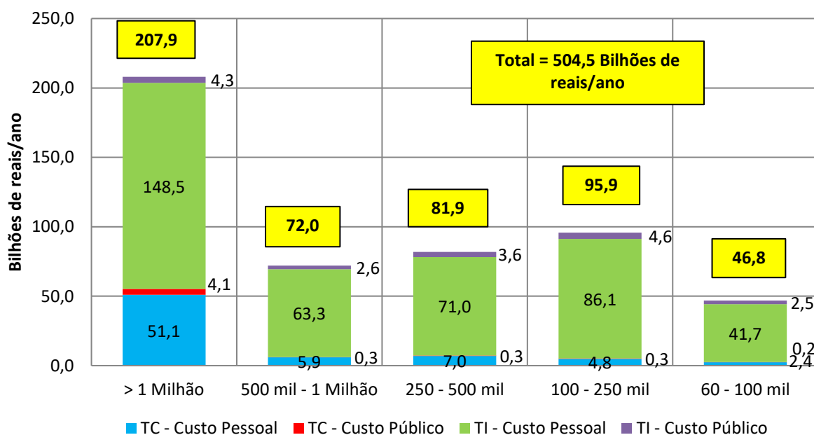
Gráfico 77 Custos anuais pessoais e públicos da mobilidade por modo de transporte e porte do município, 2023 1
