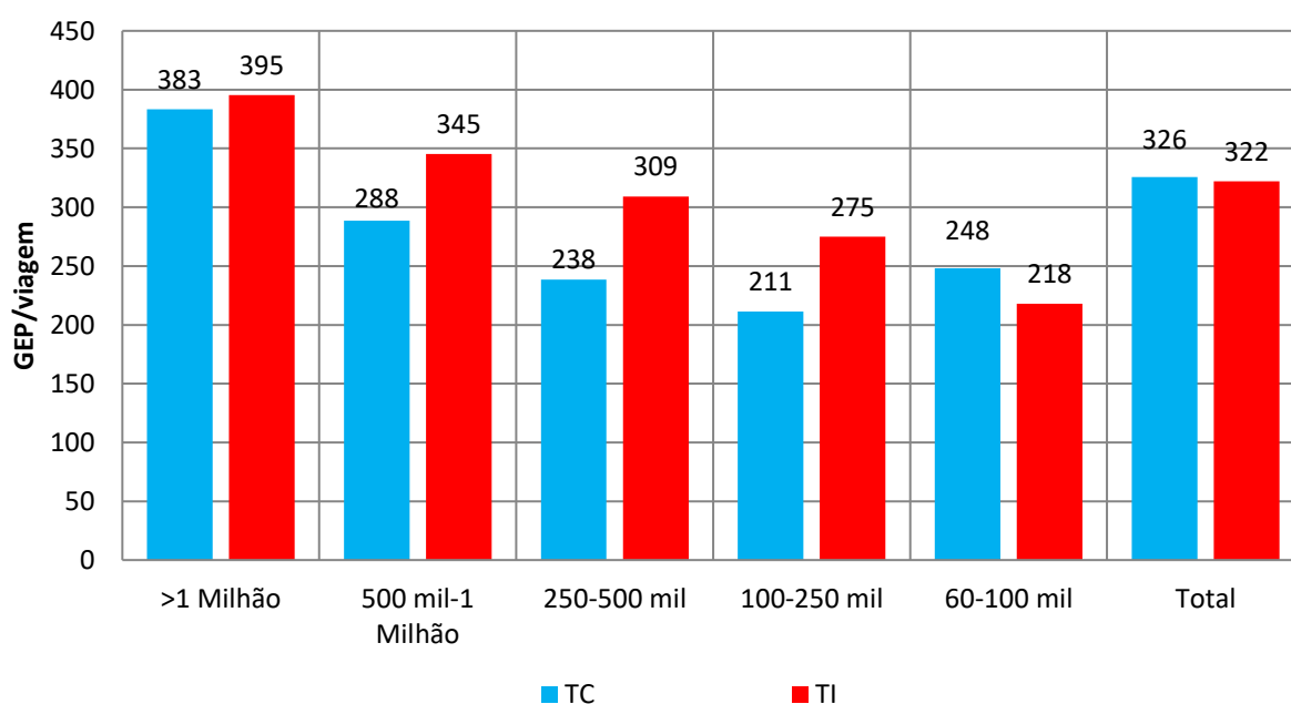
Gráfico 16 Energia gasta por viagem por modo de transporte, 2023
