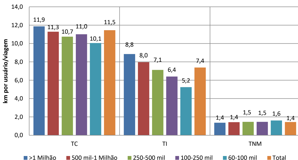
Gráfico 11 Distâncias médias das viagens por modo de transporte e porte do município, 2023
