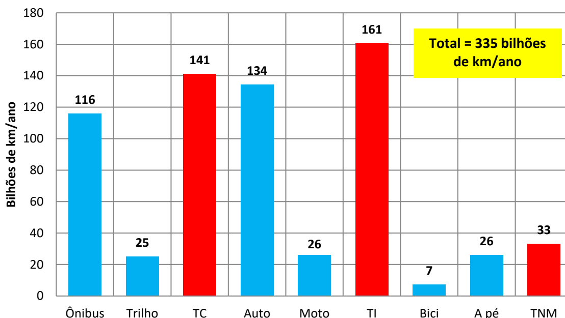
Gráfico 9 Distâncias anuais percorridas pelas pessoas por modo de transporte, 2023
