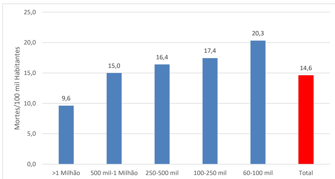
Gráfico 71 Índice de mortes por habitante e porte do município, 2023 (com dados de acidentes de 2022)
