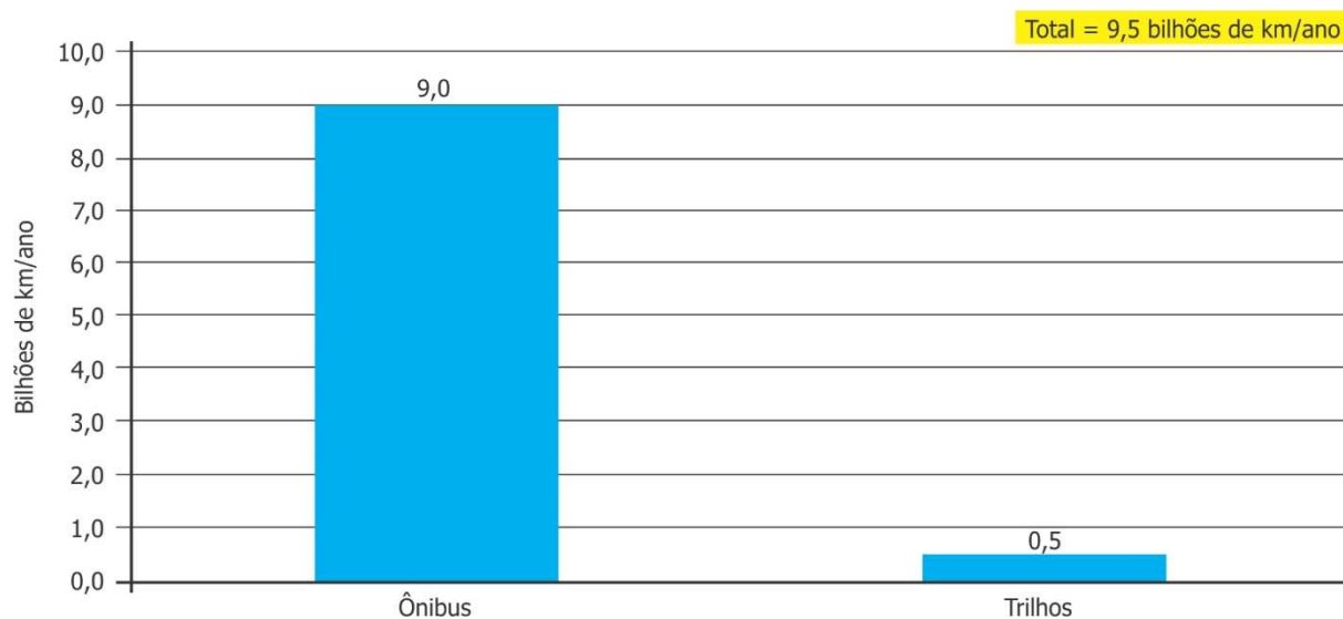
Gráfico 97 Quilometragem anual percorrida pelos veículos de transporte coletivo, 2014
