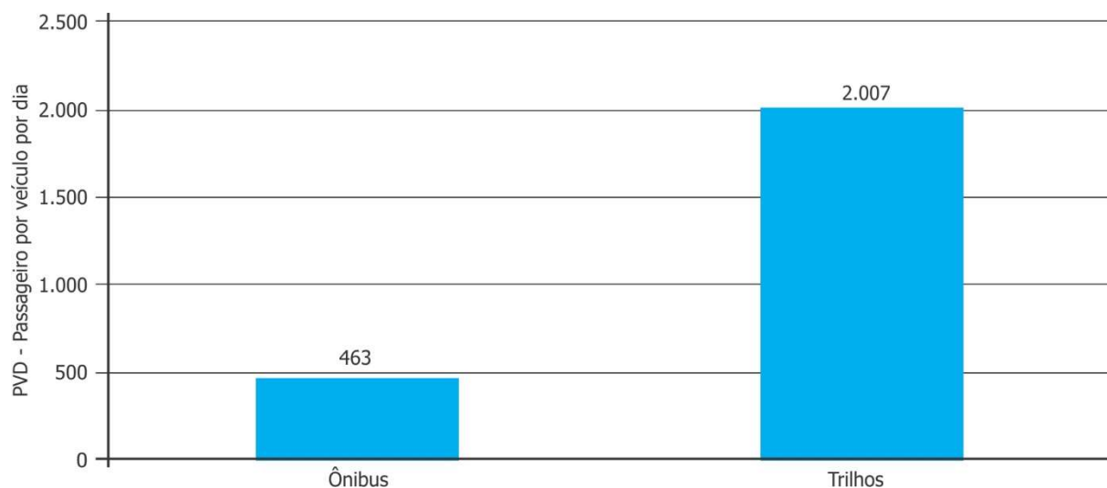
Gráfico 100 PVD 1 (passageiros por veículo por dia) do transporte coletivo, 2014
