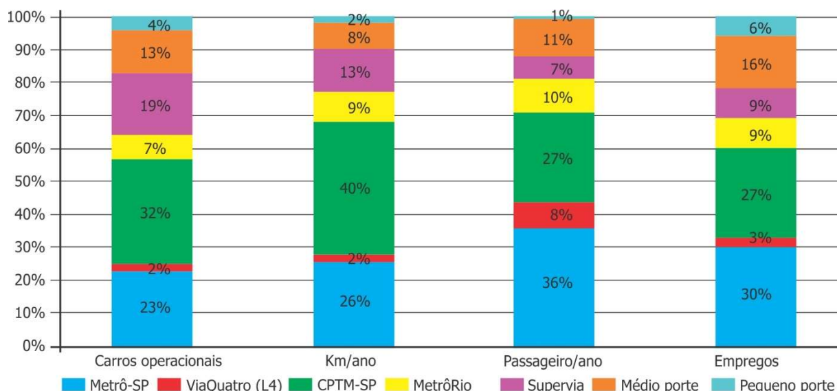
Gráfico 111 Distribuição percentual das características operacionais por sistema metroferroviário, 2014
