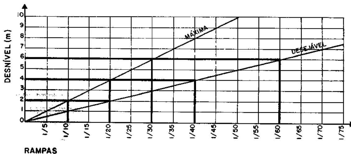
Figura 10 – Gráfico de rampas
