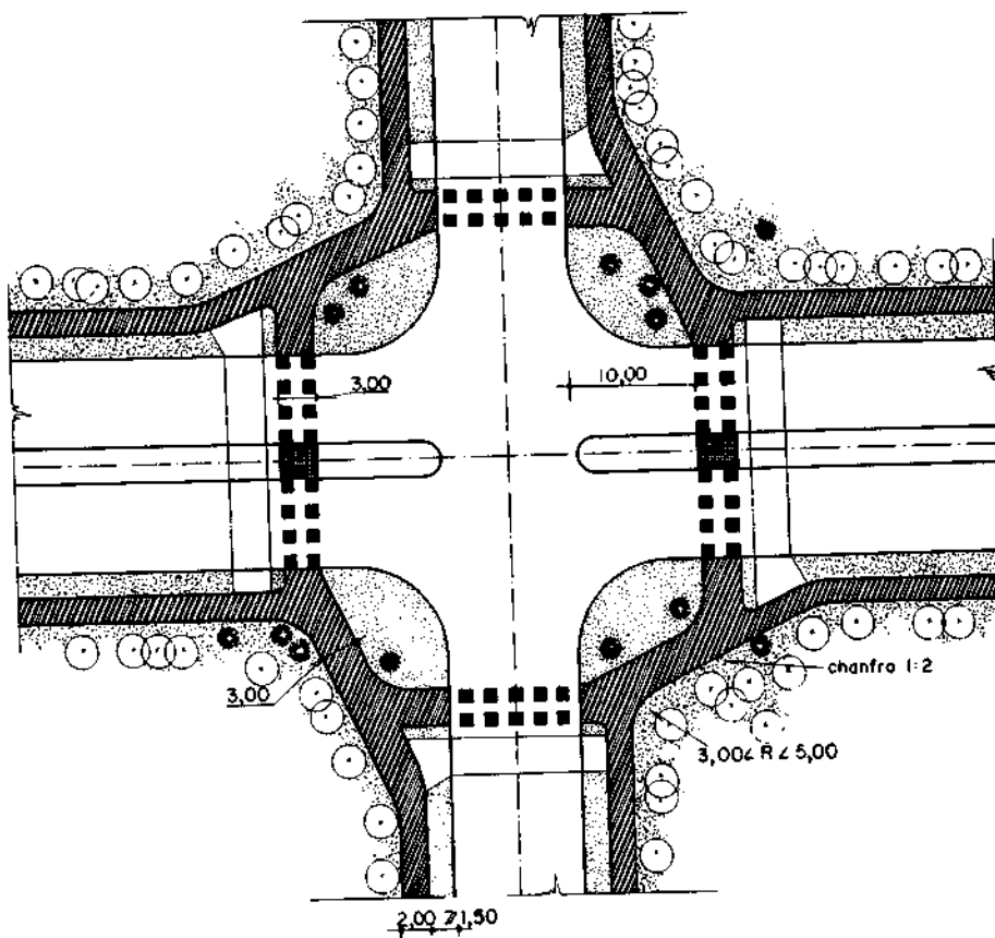
Figura 18 – Circulação canalizada num cruzamento de duas vias margeadas por ciclovias
