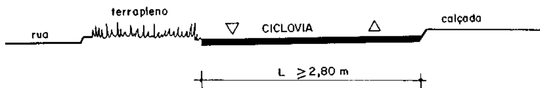
Figura 8 - Seção transversal de pista bidirecional
