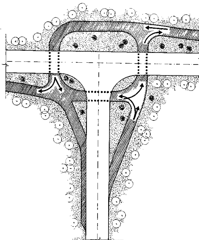
Figura 22 – Mudança de lado de uma ciclovia bidirecional, em uma interseção em T
