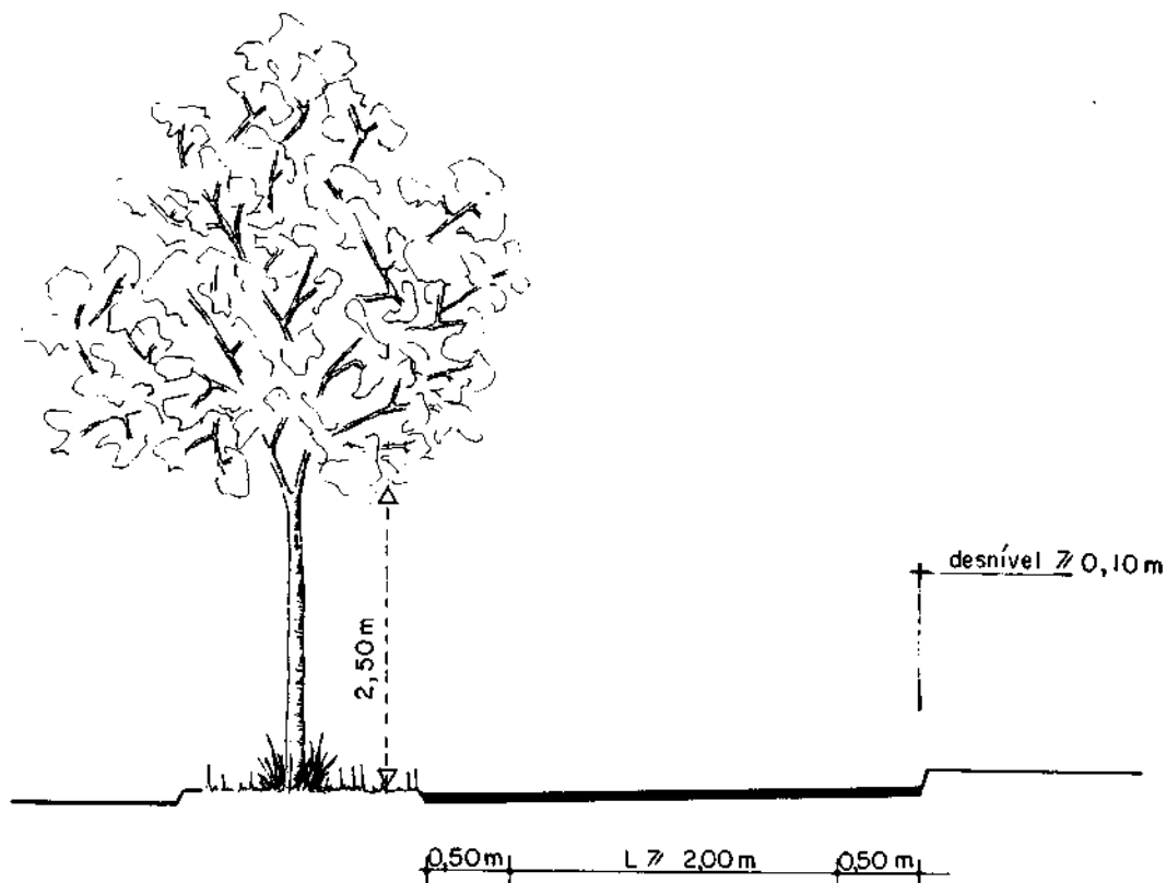
Figura 7 - Seção transversal de pista unidirecional - Caso n.º 3
