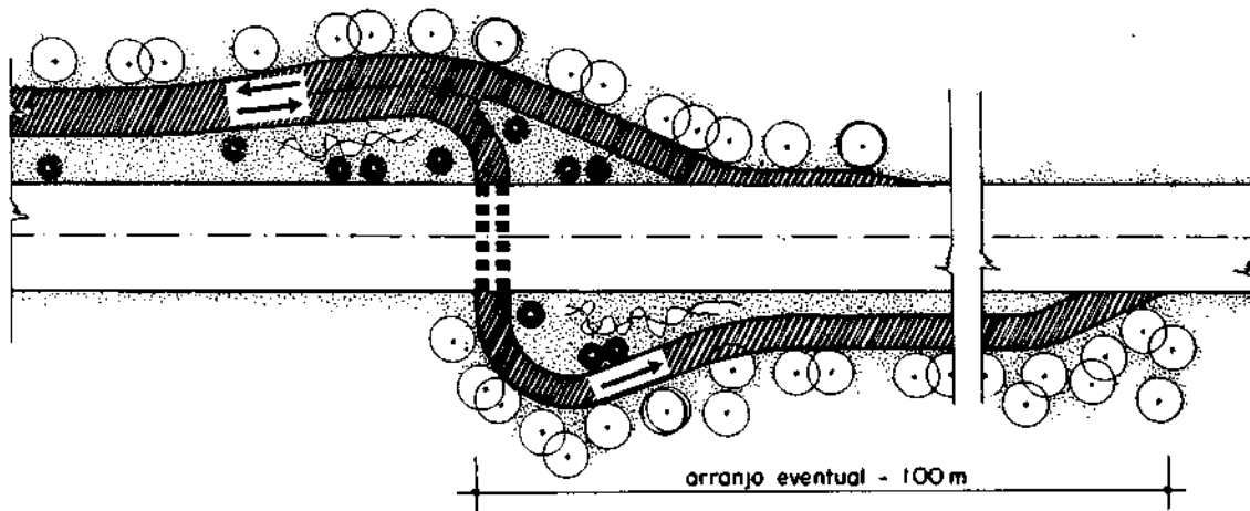
Figura 15 – Início e final de pista bidirecional – Caso n.º 2
