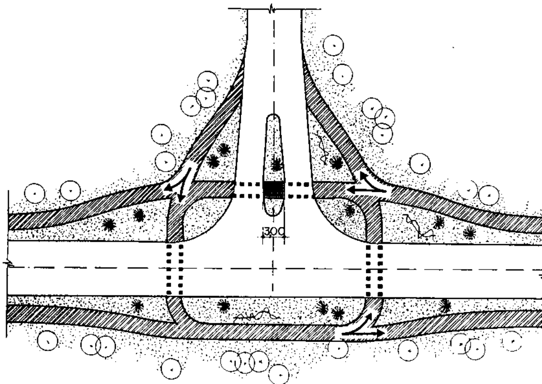
Figura 19 – Circulação canalizada em uma interseção em T
