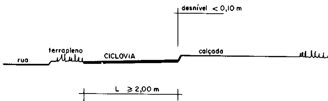
Figura 5 - Seção transversal de pista unidirecional - Caso n.º 1
