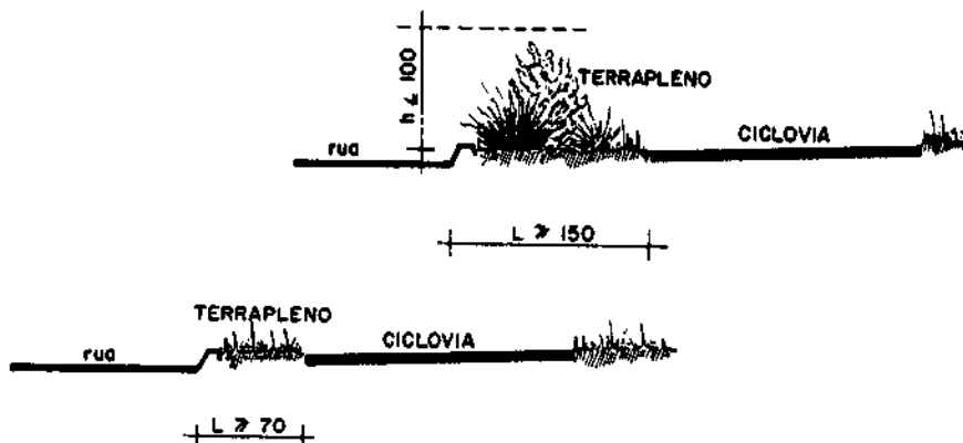
Figura 53 — Seção transversal de terraplenos
