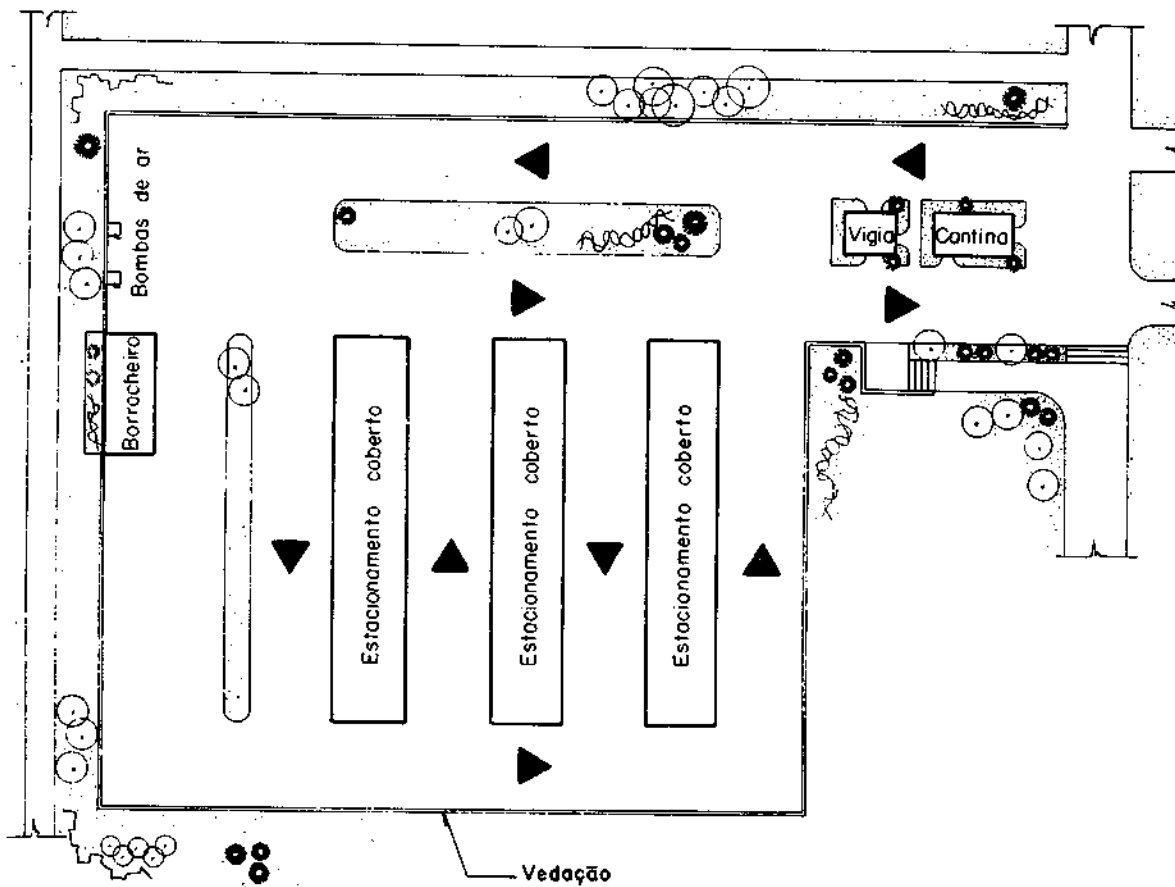
Figura 60 – Esquema de bicicletário – Caso n.º 1
