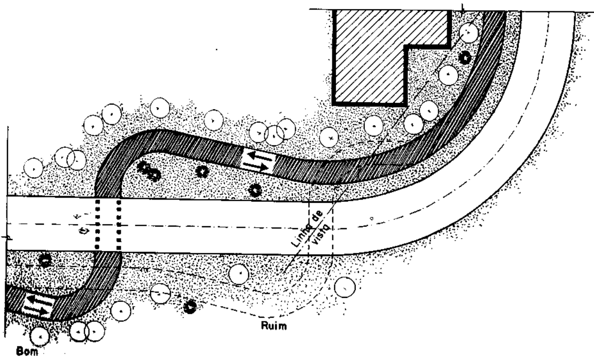
Figura 24 – Mudança de lado de uma ciclovia bidirecional, com problemas de visibilidade na aproximação de uma curva
