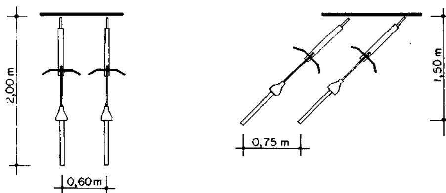
Figura 59 – Espaço requerido nos estacionamentos
