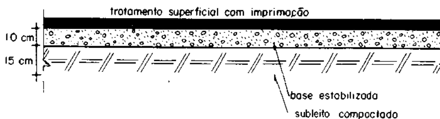
Figura 30 – Tratamento superficial simples
