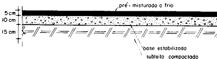
Figura 31 – Pré-misturado a frio
