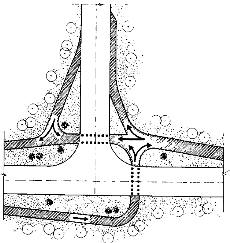
Figura 20 – Passagem de duas ciclovias unidirecionais a uma ciclovia bidirecional, em uma interseção em T
