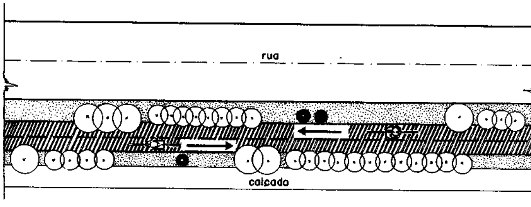
Figura 55 – Sombreamento nas ciclovias com plantações alternadas
