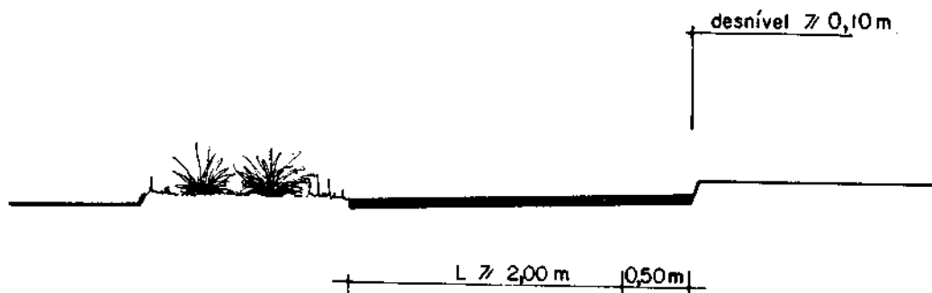
Figura 6 - Seção transversal de pista unidirecional - Caso n.º 2
