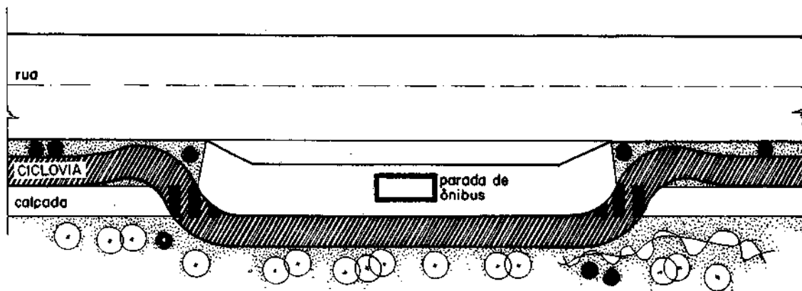
Figura 16 – Ciclovias em parada de ônibus
