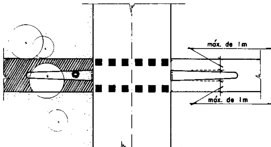
Ilha direcional na entrada de ciclovia
