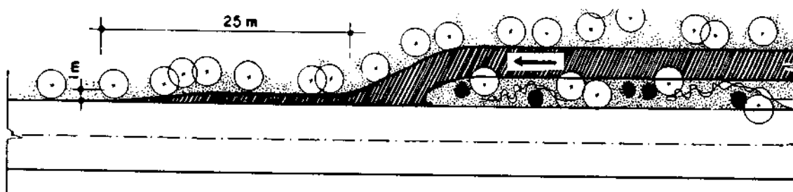
Figura 13 – Final de pista unidirecional – Caso n.º 2
