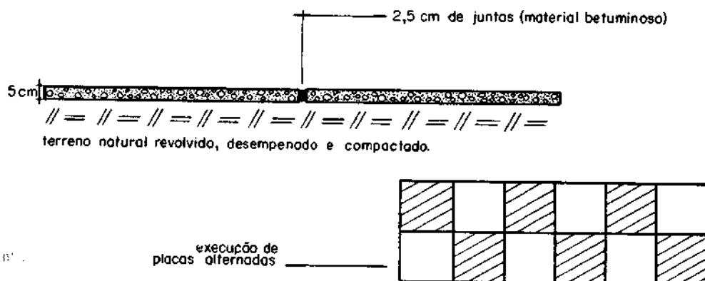
Figura 27 - Concreto moldado no local
