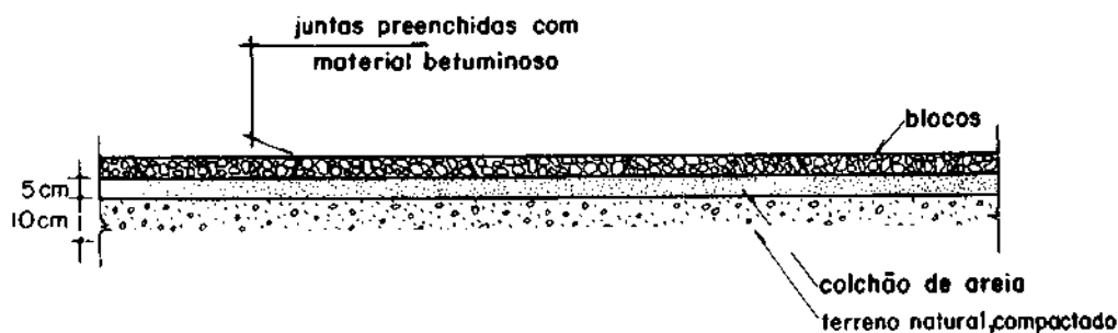
Figura 29 – Blocos pré-moldados de concreto
