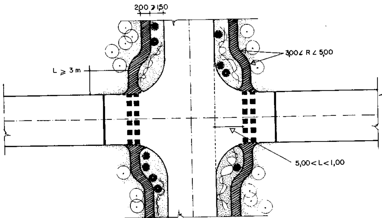
Figura 17 – Circulação canalizada em um cruzamento entre uma via com ciclovias unidirecionais e uma via sem ciclovias
