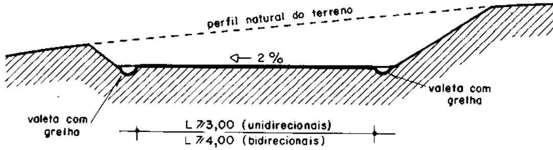
Figura 35 — Drenagem em um corte simples
