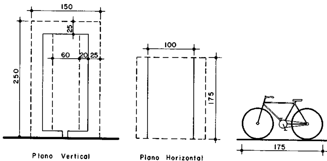
Figura 1 -- Espaço útil de um ciclista (em cm)
