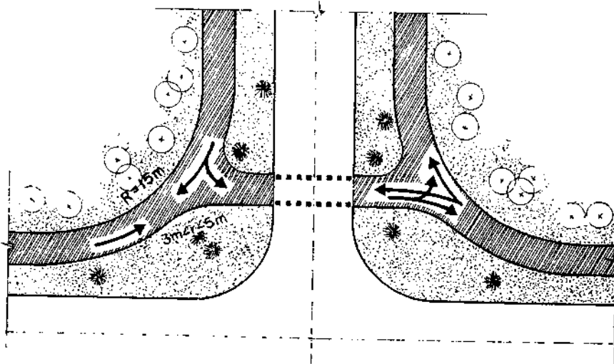
Figura 21 – Interseção de uma rua margeada de ciclovia bidirecional, com uma rua margeada por duas ciclovias unidirecionais
