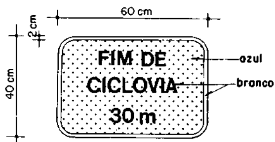
Figura 45 – Placa I-27: Aproximação de final de ciclovía (dirigida aos ciclistas)
