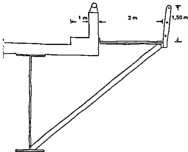
Passarela para bicicletas, em alargamento de pontes e viadutos
