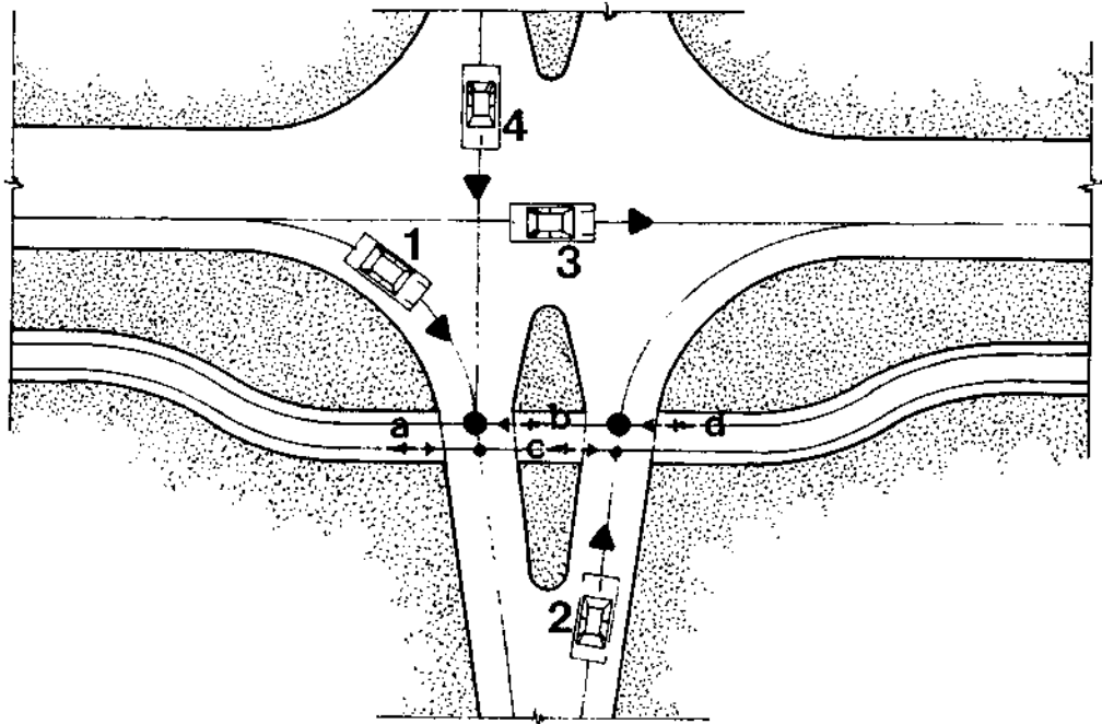
Problemas de segurança em uma travessia de pista bidirecional
