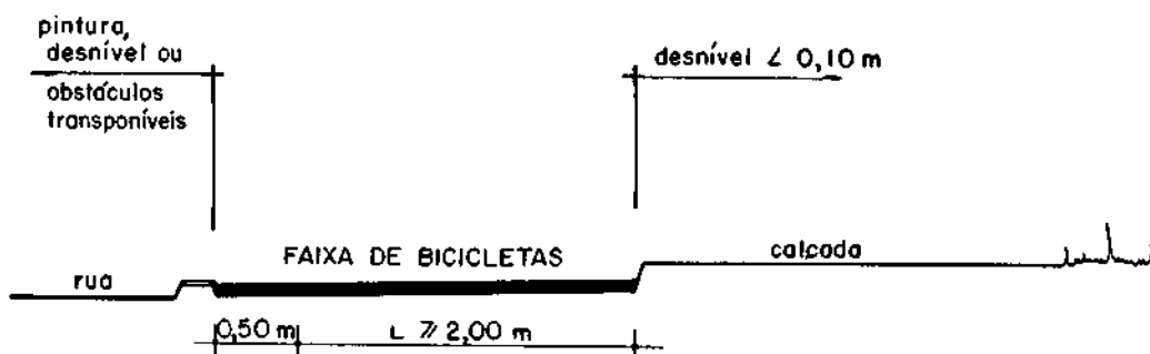
Figura 9 – Seção transversal de faixa de ciclistas
