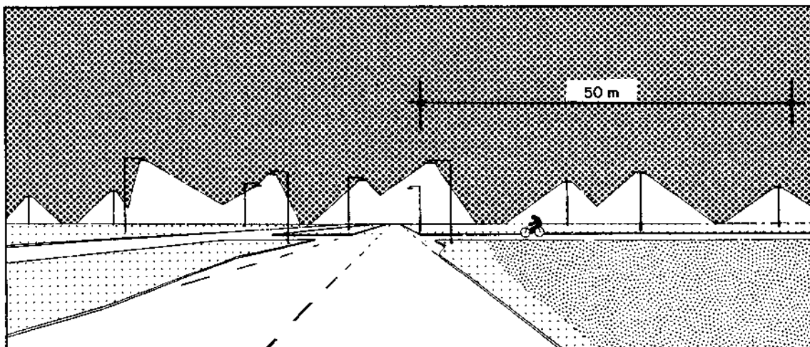
Figura 58 – Iluminação na aproximação de uma travessia de ciclistas
