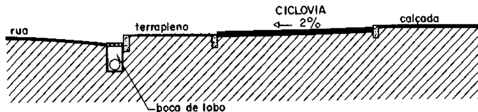
Figura 32 — Inclinação lateral de uma ciclovia
