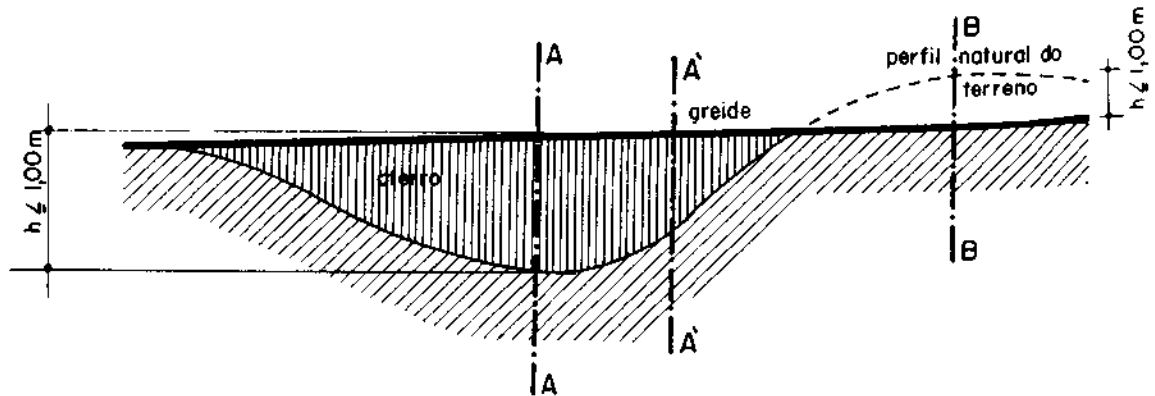
Figura 33 – Perfil longitudinal do terreno natural e do greide da ciclovia
