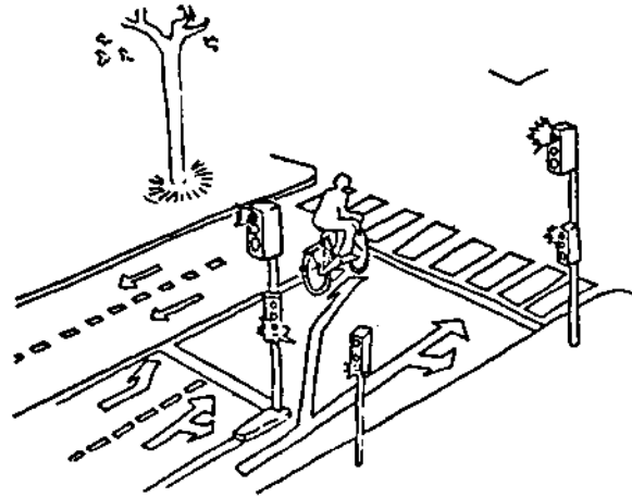
Conversão à esquerda, com área de acumulação para bicicletas e semáforos para ciclistas (Holanda)
