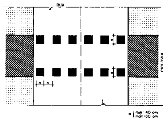
Figura 48 — Travessia em nível para ciclistas
