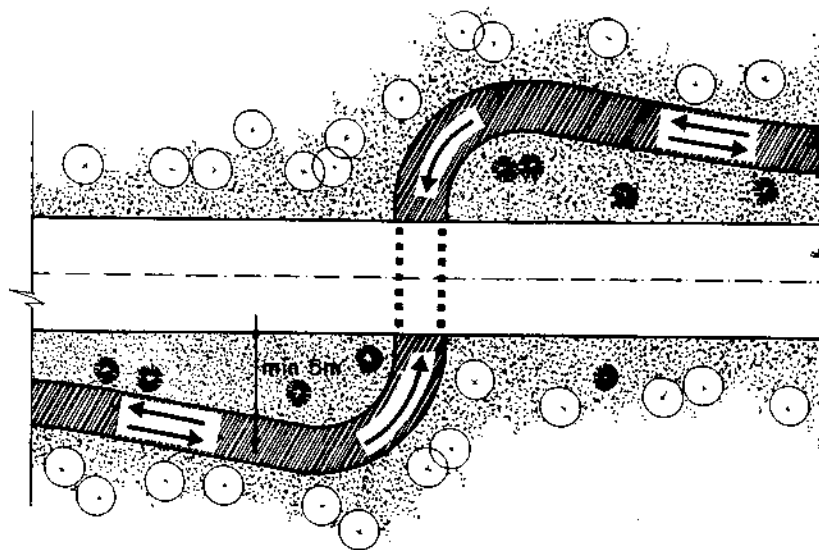
Figura 23 – Mudança de lado de uma ciclovia bidirecional
