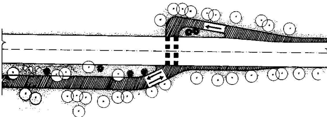
Figura 14 – Início e final de pista bidirecional – Caso n.º 1
