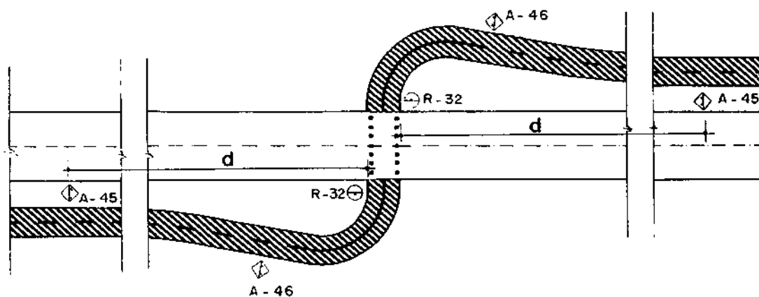
Figura 46 – Sinalização vertical em uma mudança de lado
