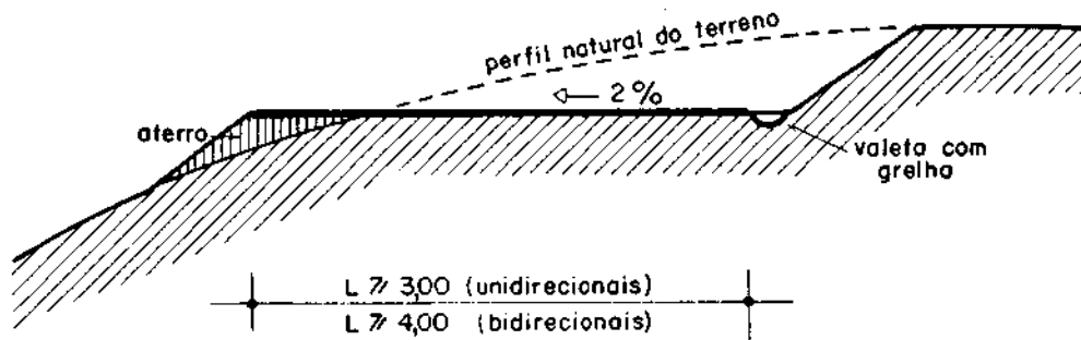
Figura 36 — Drenagem em um corte com compensação
