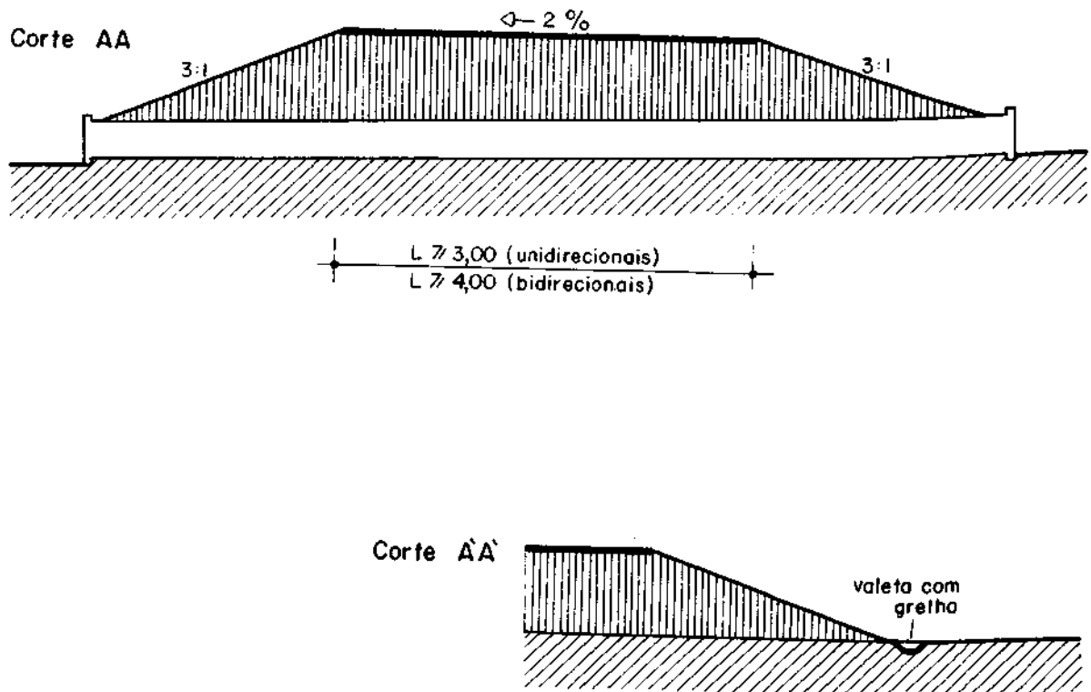
Figura 34 – Drenagem nos aterros
